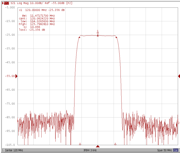
Attenuation Fo±7.5MHz
