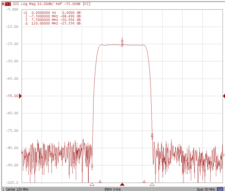
Attenuation Fo±7.5MHz
